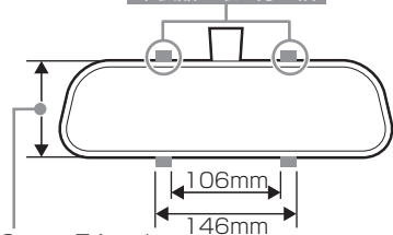
本製品の取り付け幅
