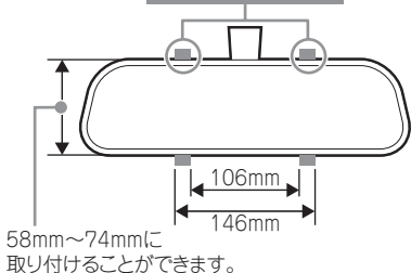
本製品の取り付け幅
