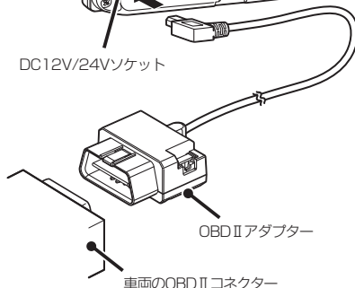
車両のOBD II コネクター
