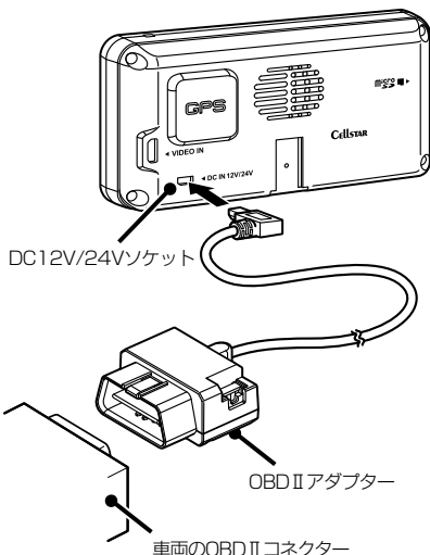
車両のOBD II コネクター
